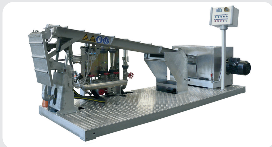
Unterwasser-Stranggranulator
