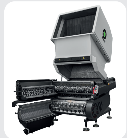
Schredder
