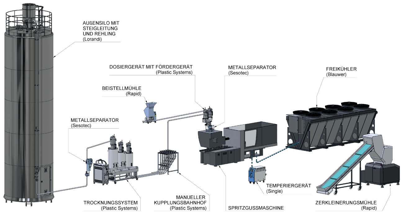
Spritzguss-Schema
